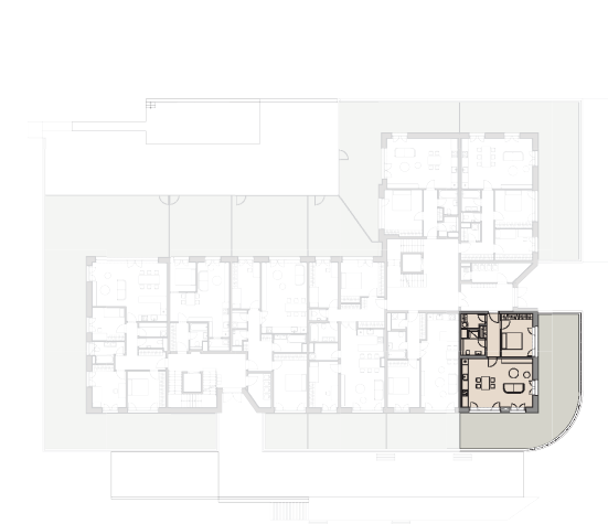
BYTOVÝ DŮM G1 - 1.NP
